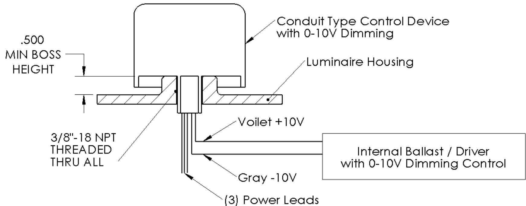
External Conduit Style Control
